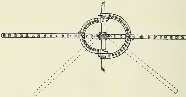
Fig. 163. Winkelmesser von GUTSCH.
